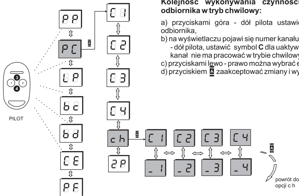
Rys.14. Procedura zmiany trybu chwilowego
