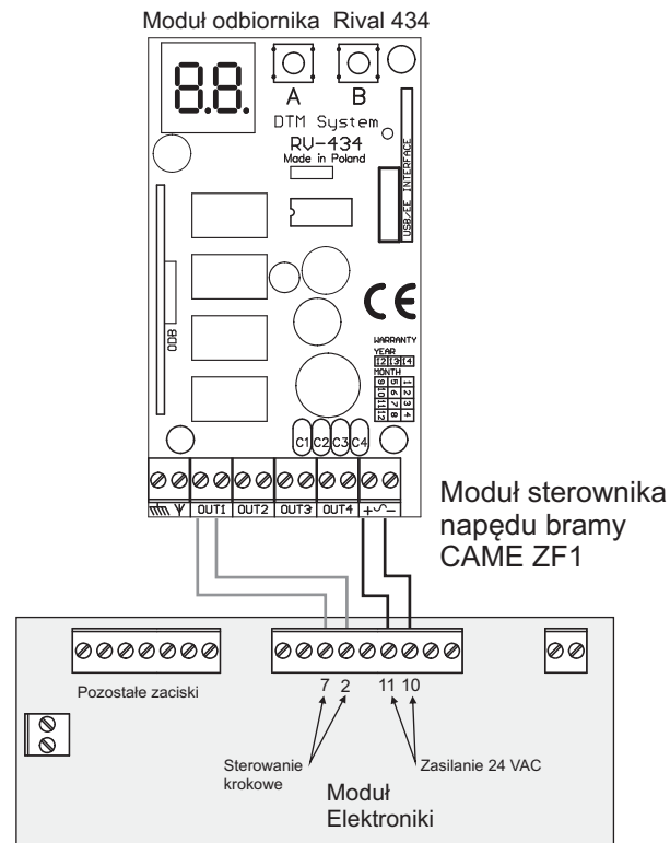
Schemat 2. Przykład połączenia sterownika napędu bramy CAME ZF1 z odbiornikiem Rival 434.
