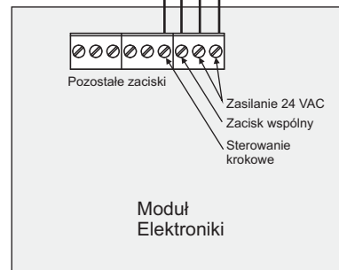
Schemat 4. Przykład połączenia sterownika napędu bramy NICE z odbiornikiem Rival 434.
