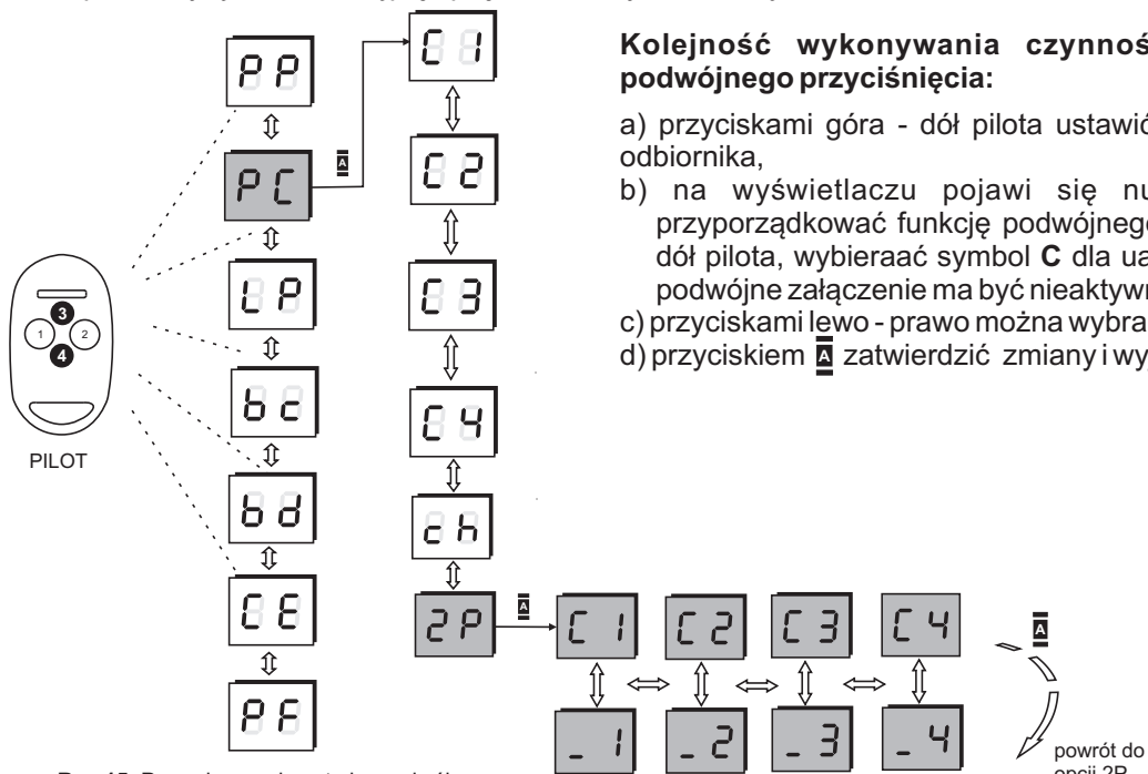
Rys.15. Procedura zmiany trybu podwójnego przyciśnięcia
