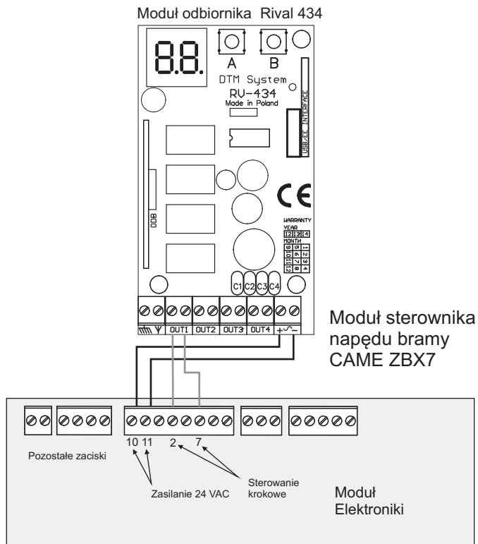
Schemat 1. Przykład połączenia sterownika napędu bramy CAME ZBX7 z odbiornikiem Rival 434.
