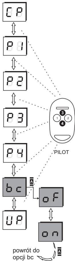
Rys.11. Procedura blokady prostego dopisywania pilota
