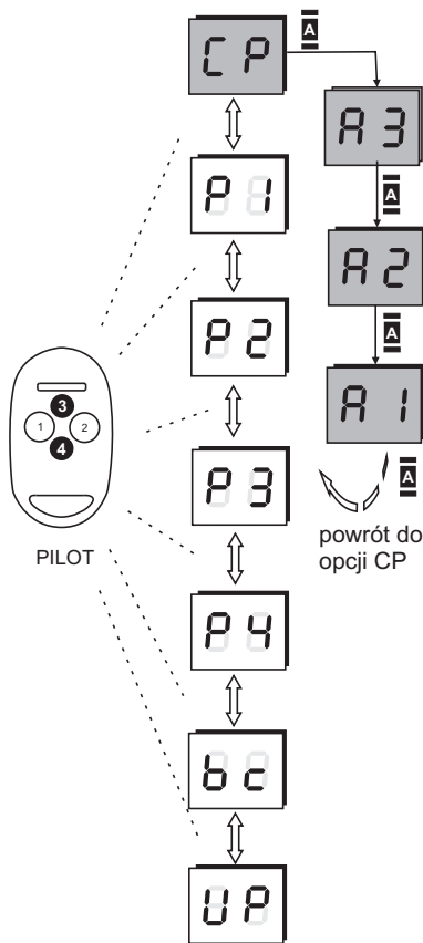
Rys.9. Procedura kopiowania nastaw pilota
