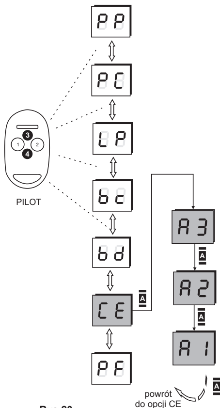
Rys.20 Klonowanie pamięci odbiornika
