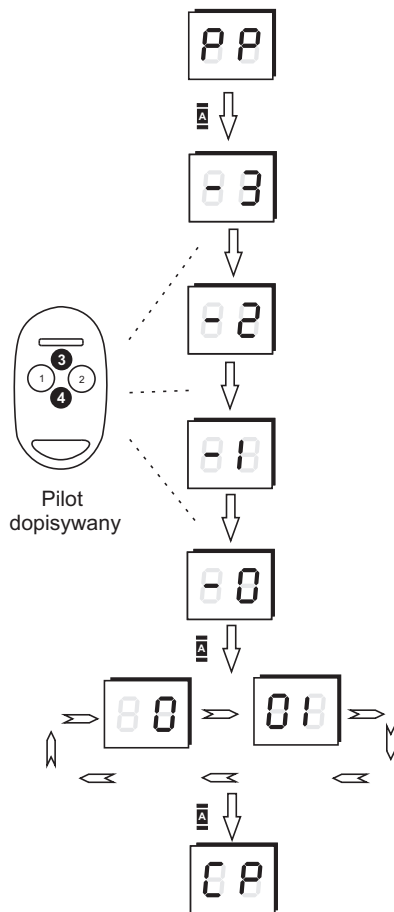
Rys.7. Procedura dopisywania nowego pilota.
