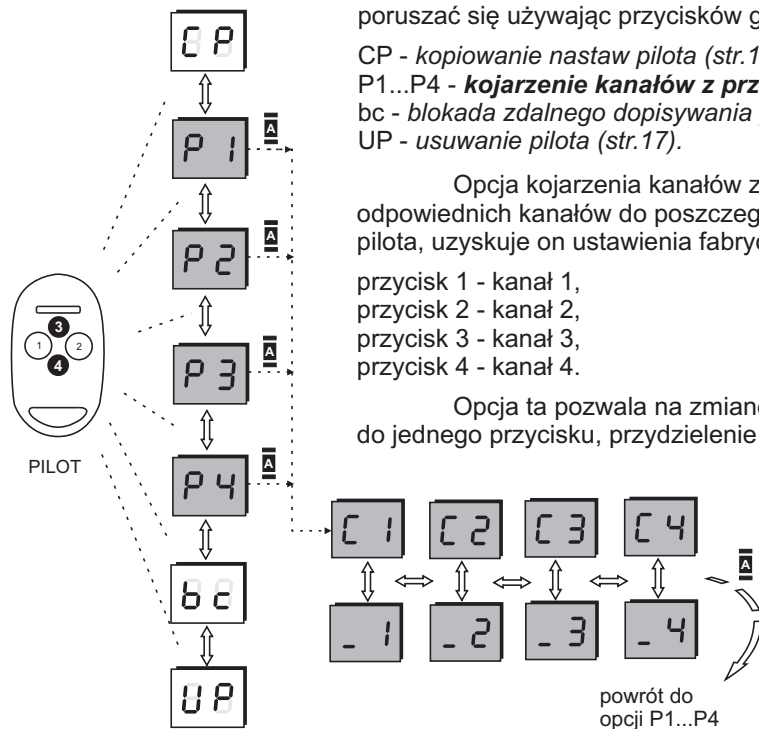
Rys.10. Procedura kojarzenia kanałów z przyciskami pilota
