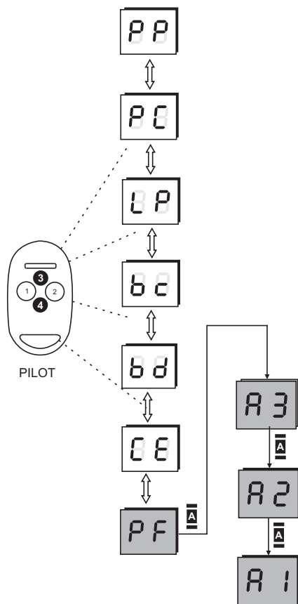
rys.21 Przywrócenie pamięci fabrycznej odbiornika.
