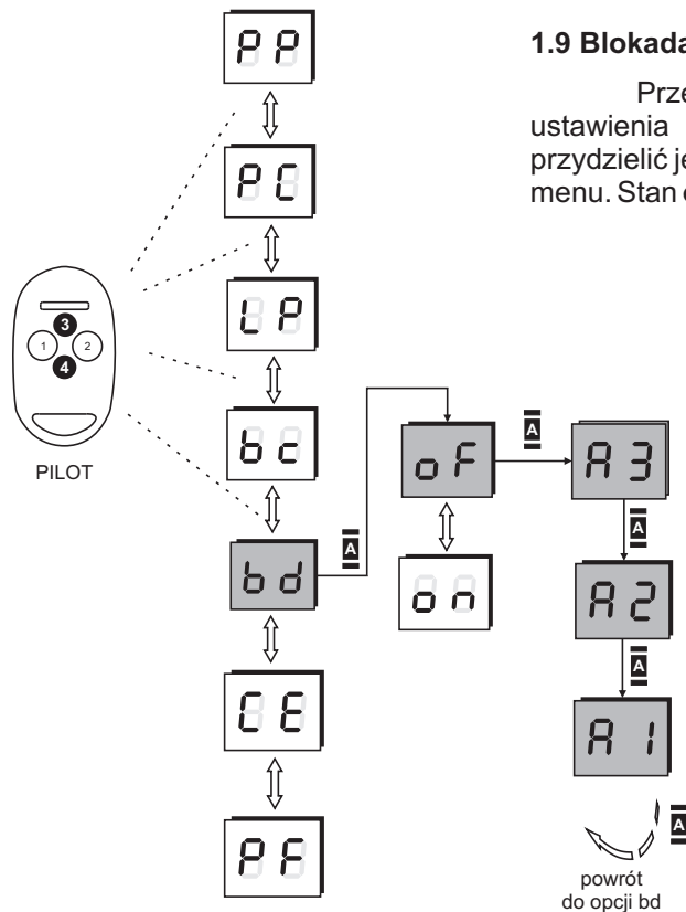
Rys.18. Procedura wyłączenia blokady menu (wprowadzania kodu PIN)
