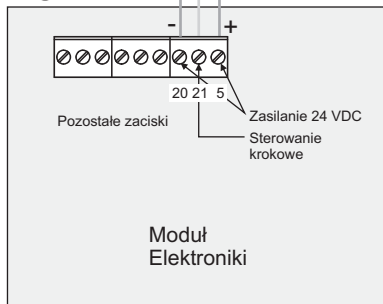
Schemat 3. Przykład połączenia sterownika napędu bramy Hormann z odbiornikiem Rival 434.
