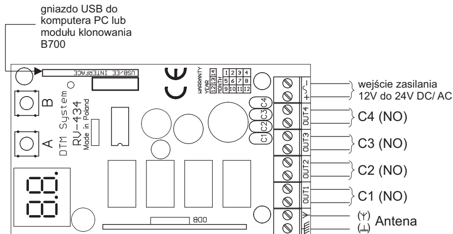
rys 1. Schemat elektryczny instalacji odbiornika Rival 434
