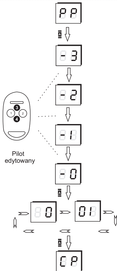
Rys.8. Procedura edycji nowego pilota
