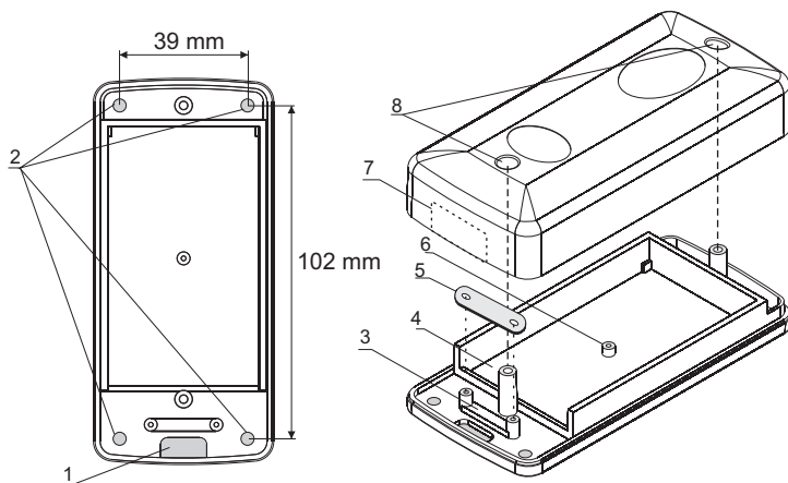
rys.3 Widok obudowy odbiornika Rival 434.
