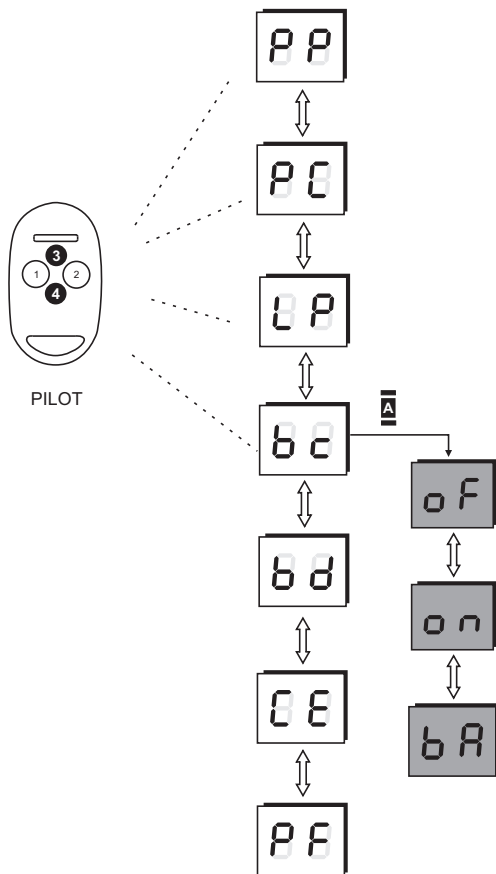
Rys.17. Procedura włączenia/wyłączenia globalnej blokady prostego dopisywania pilotów
